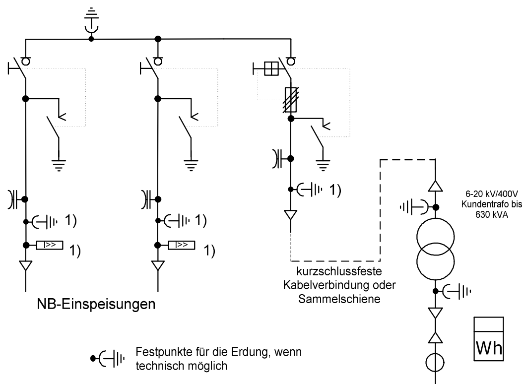
Bild 1 Baustromstation mit niederspannungsseitiger Messung
