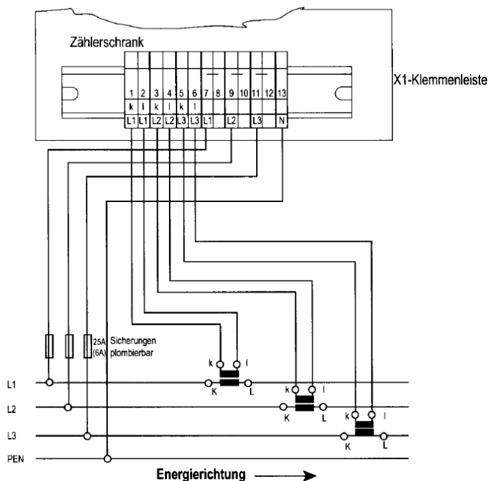
Schaltbild für den Anschluss der Strom- und Spannungsmessleitungen
