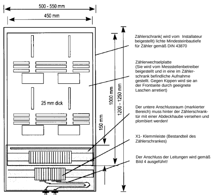
Prinzip- und Maßbild des Zählerschranks bzw. der Zählerwechselplatte
