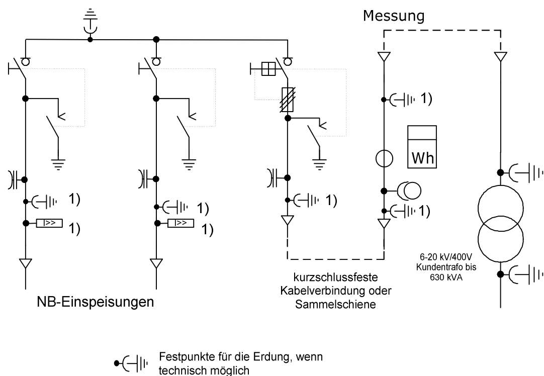
Bild 2 Baustromstation mit mittelspannungsseitiger Messung
